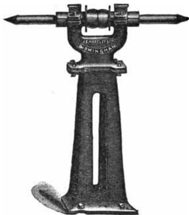
FIG. 38. POLISHING LATHR.
